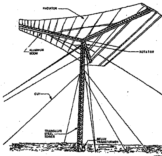
Rotatable log-periodic antenna.
